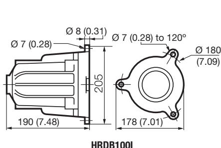
HRDB100I
