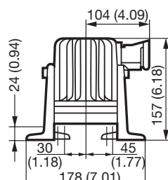
HRDC020ZE
